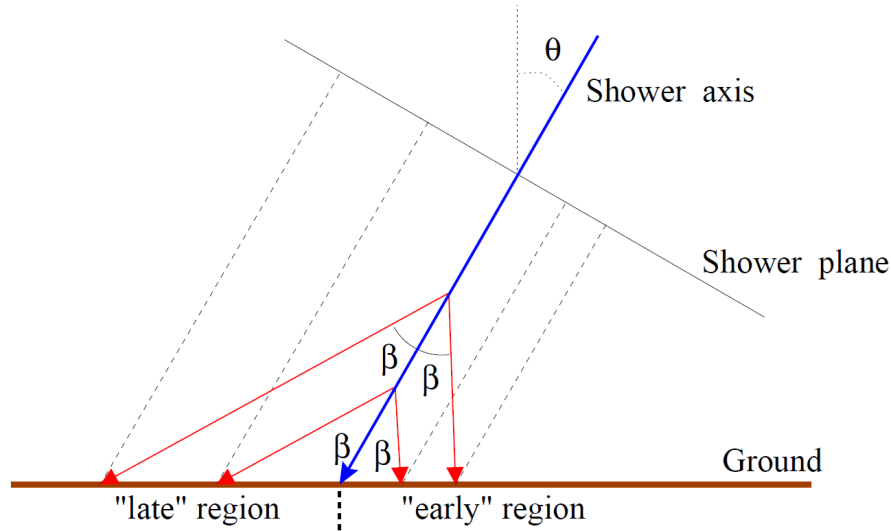
Figura 3.5: Esquema geométrico de cómo es la dispersión de las partículas con el ángulo de emisión respecto al eje de la lluvia \alpha (en la imagen llamado \beta ). Se ve que para un mismo ángulo de emisión, se alcanza una región mucho más tardía que temprana.
