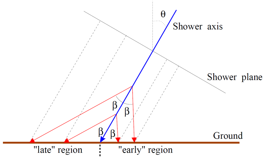
Figura 3.6: Esquema geométrico de cómo es la dispersión de las partículas con el ángulo de emisión respecto al eje de la lluvia \alpha (en la imagen llamado \beta ). Se ve que para un mismo ángulo de emisión, se alcanza una región mucho más tardía que temprana.
