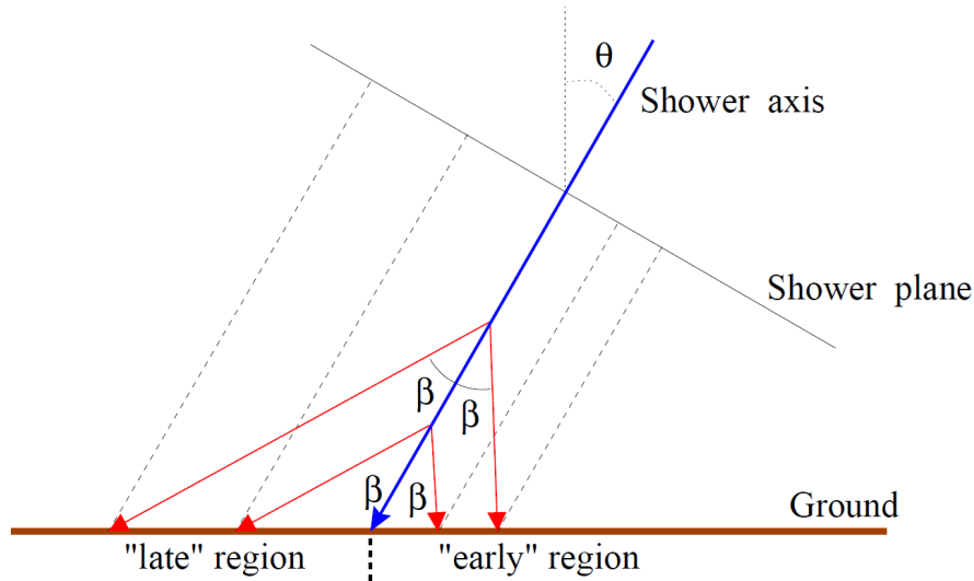
Figura 3.4: Esquema geométrico de cómo es la dispersión de las partículas con el ángulo de emisión respecto al eje de la lluvia \alpha (en la imagen llamado \beta ). Se ve que para un mismo ángulo de emisión, se alcanza una región mucho más tardía que temprana.
